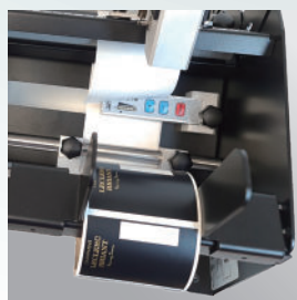
Ultraschall-Etiketten-Sensor
